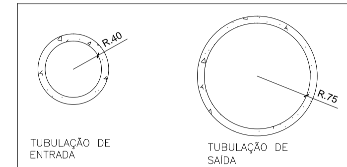
DETALHE TUBULAÇÃO DE CANALIZAÇÃO DE ÁGUA Esc.:1/50
