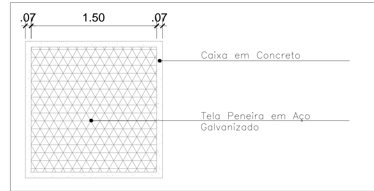
DETALHE DO LADRÃO COM GRADIL Esc.:1/25
