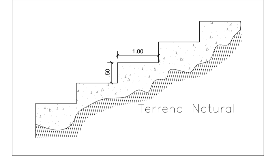
DETALHE ESCADA DISSIPADOR DE ENERGIA Esc.:1/50
